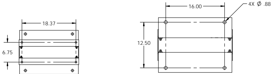
SECTION B-B SCALE 1 : 8
