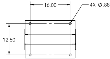
SECTION B-B SCALE 1 : 10
